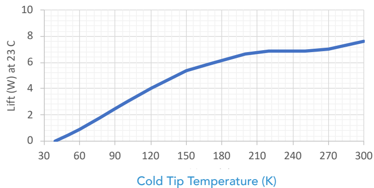
DS Mini Nominal Performance
